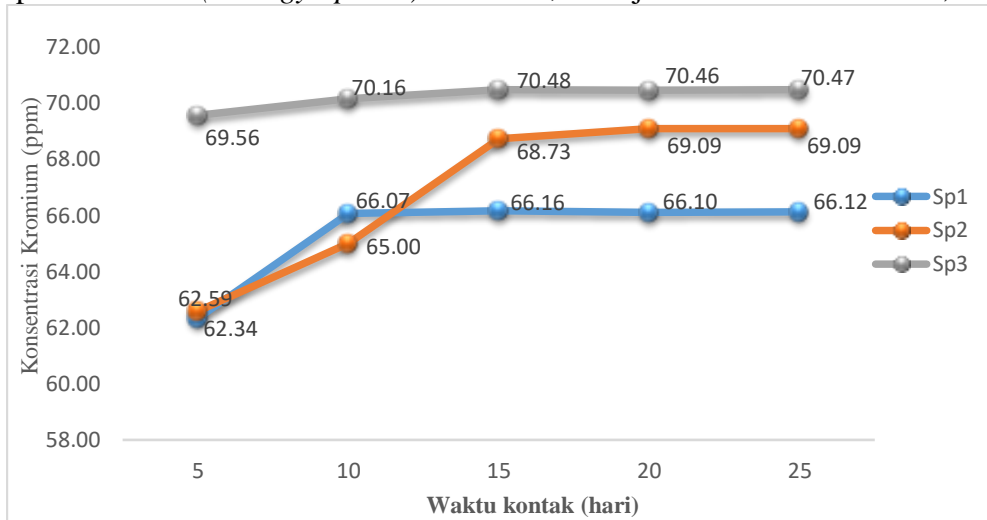
Gambar 1. Tingkat Serapan Kromium oleh Simbiosis Sponge Petrosia (Strongylophore) Corticata Berdasarkan Waktu Kontak
