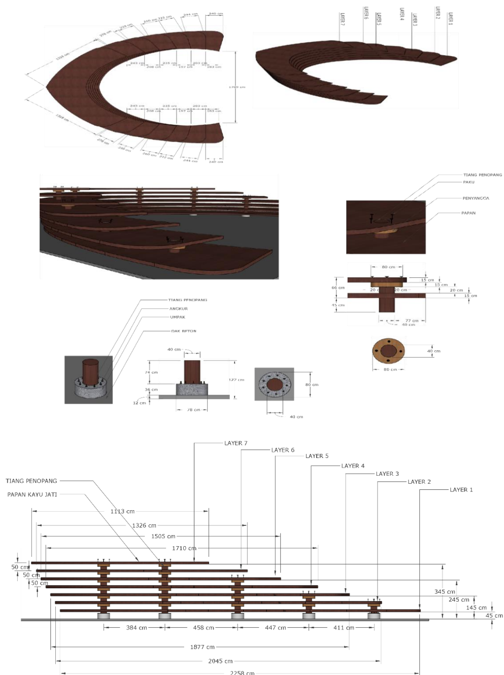
Gambar 2. Detail pendekatan fasad lamba'na Sumber: Hasil Desain (2025)
