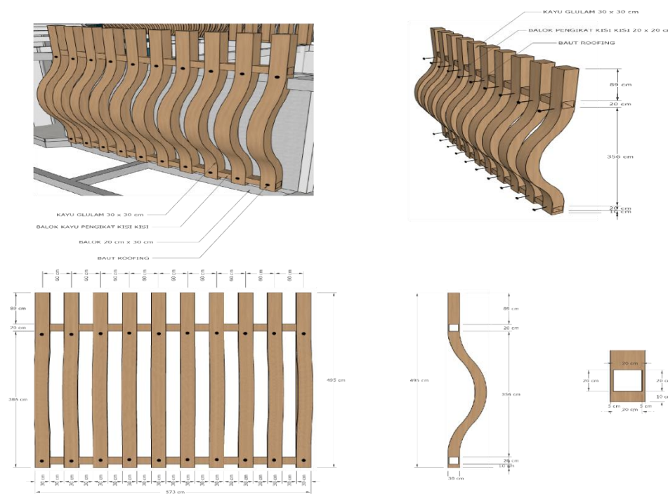
Gambar 3. Detail pendekatan fasad Uai Sumber: Hasil Desain (2025)
